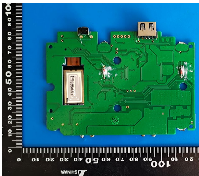
Fig. 6 – Back view of PCM 表6 – PCM 反面视图
