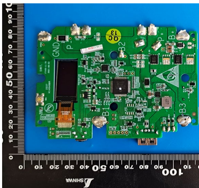
Fig. 5 – Front view of PCM 表5 – PCM 正面视图
