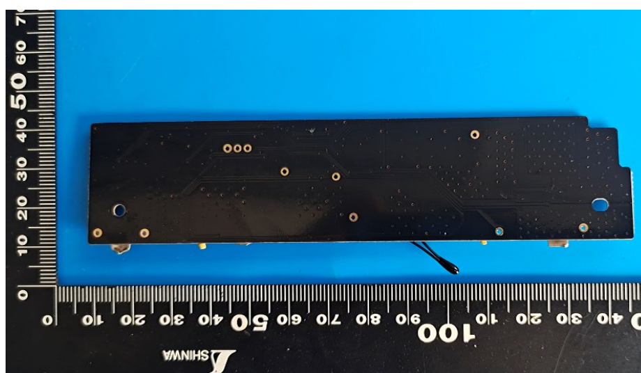
Fig. 6 – Back view of PCM 表6 – PCM 反面视图
