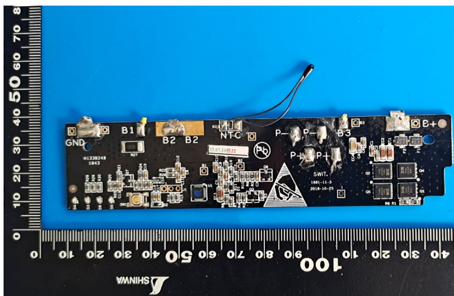
Fig. 5 – Front view of PCM 表5 – PCM 正面视图
